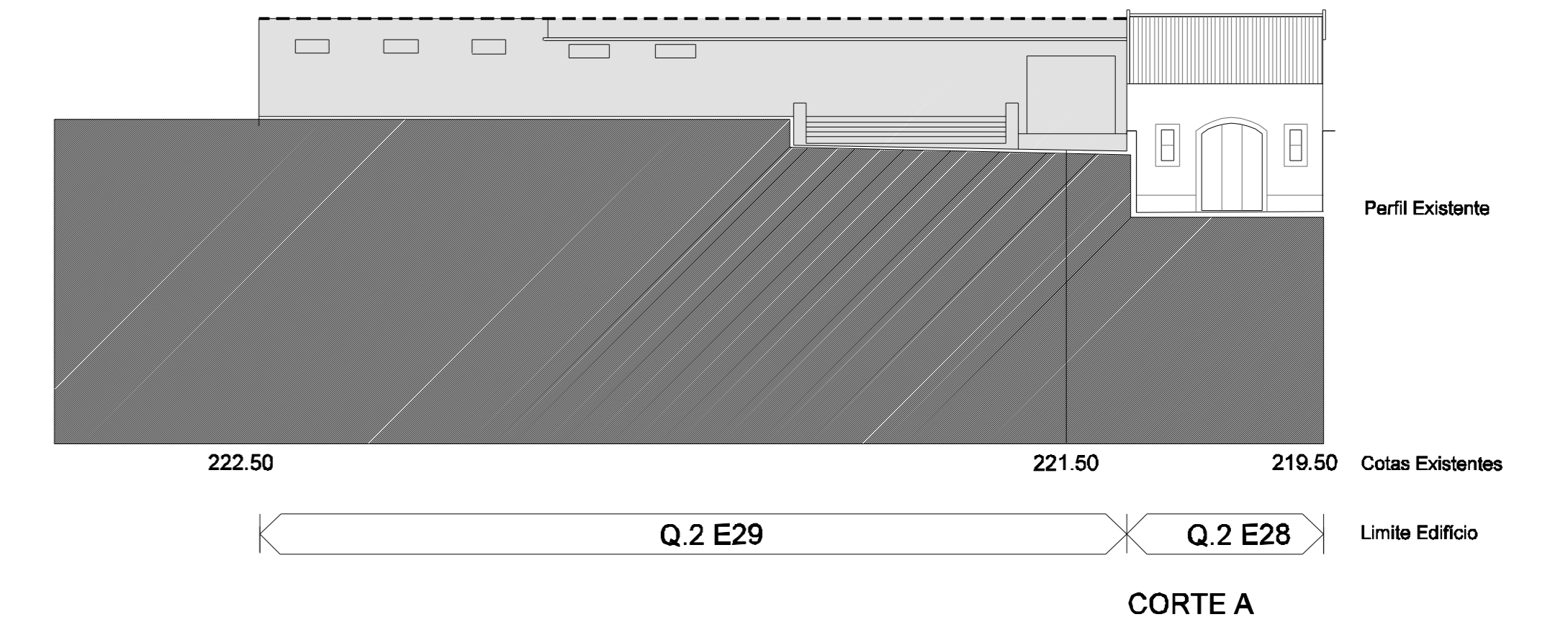
CORTE A
