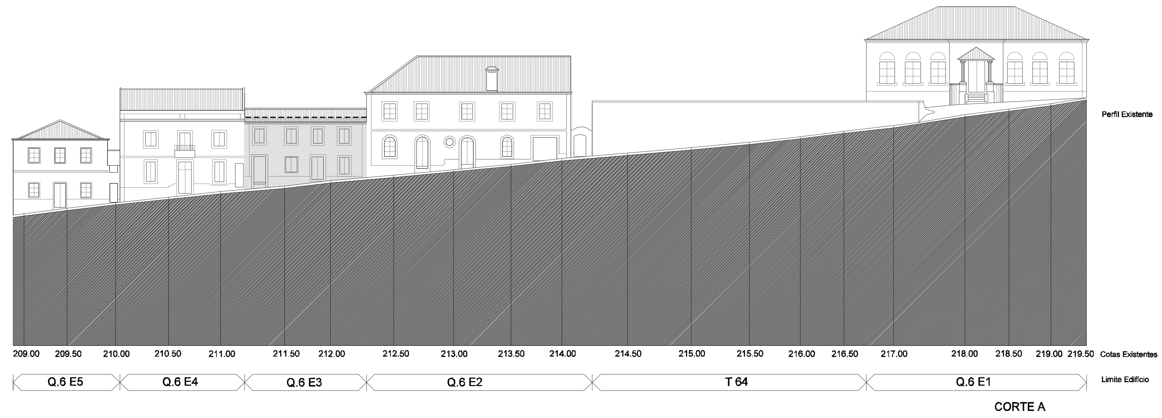
CORTE A
