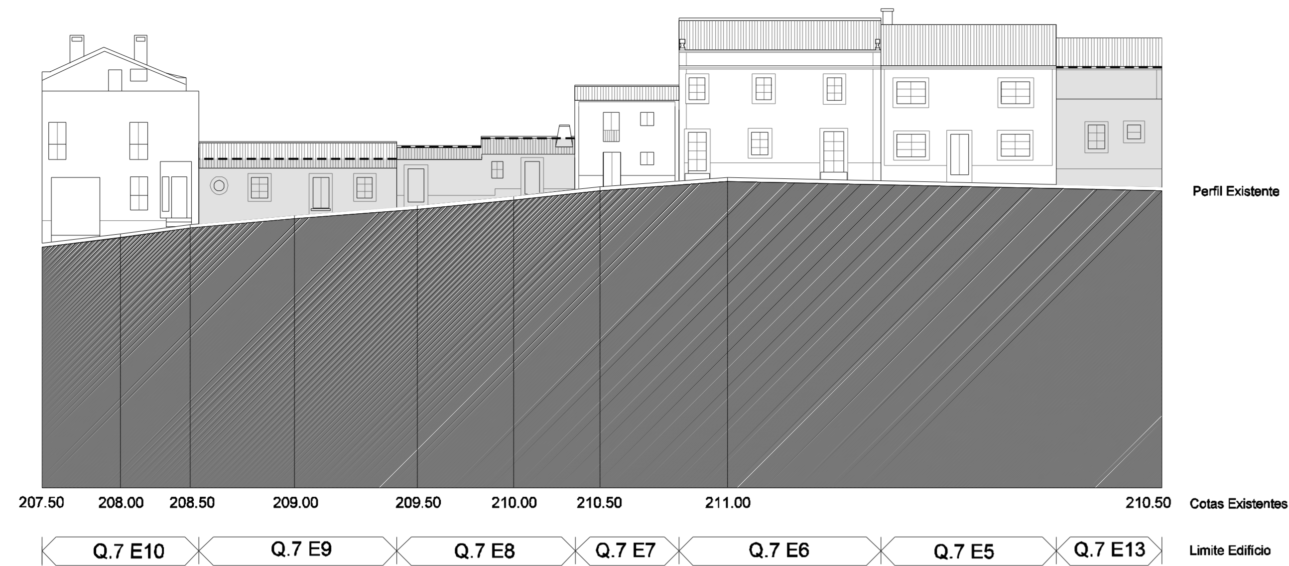
CORTE A
