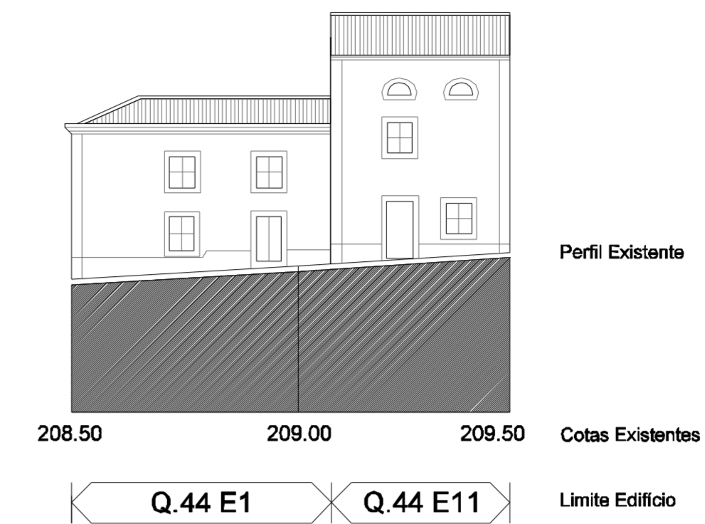
CORTE A
