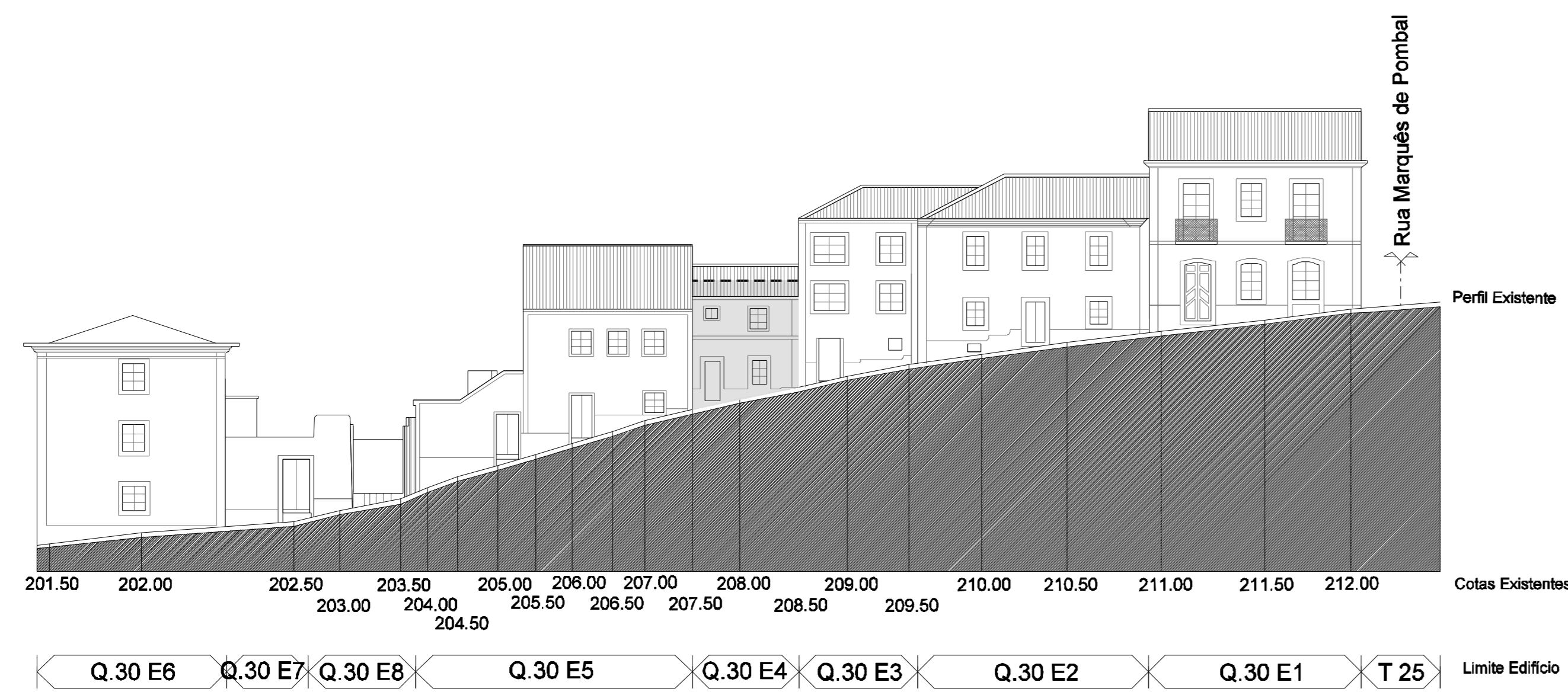
CORTE A
